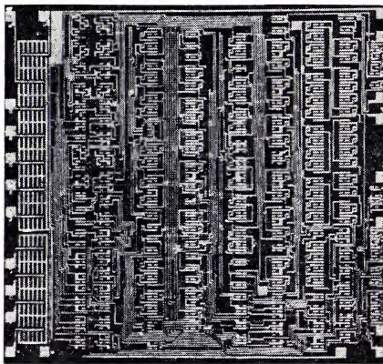
Рис. 4. Большая интегральная микросхема для электронных часов. В кристалле кремния с активной площадью около 3 \text{ м}^2 создано 1438 n - и p -канальных полевых транзисторов, образующих посредством двухслойной системы связей микро-ЭВМ, к-рая ведёт отсчёт текущего времени суток (секунд, минут, часов), дней недели, дат; расходуемая мощность не более 10 \text{ мвт} .
